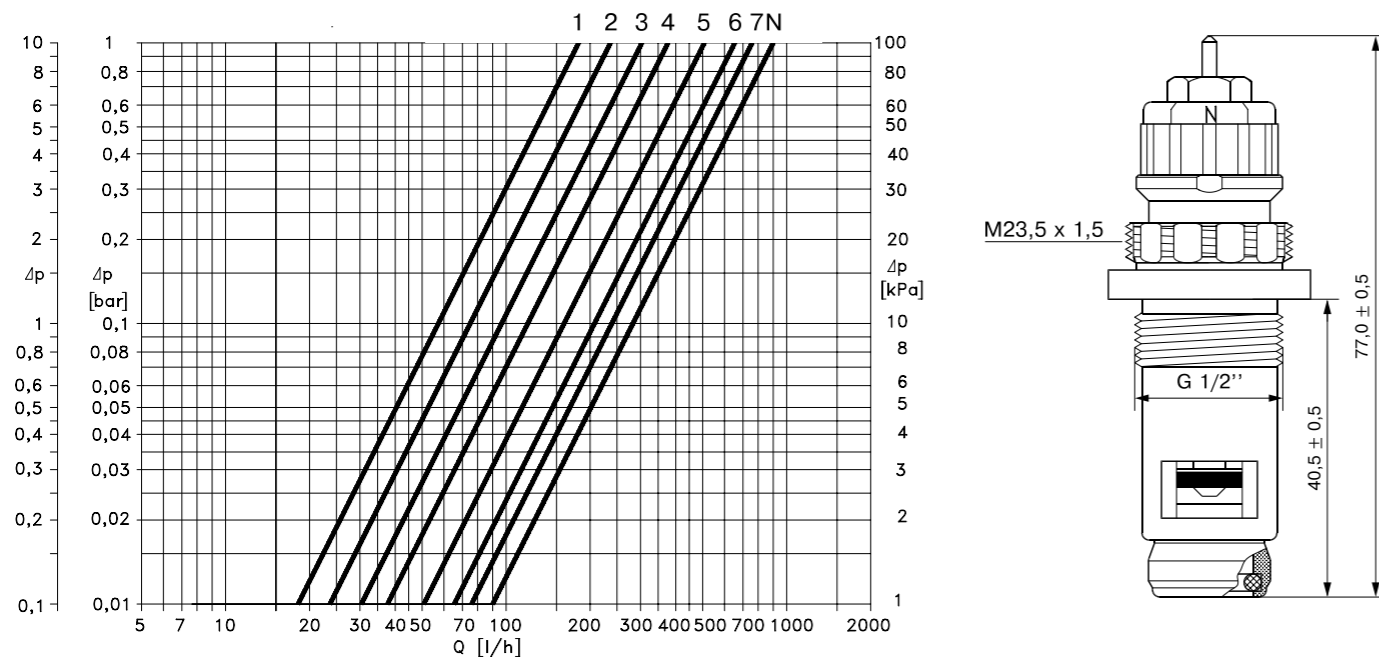
Диаграммы для термостатического клапана Danfoss 013G1382 без узла нижнего подключения при 2 °С
