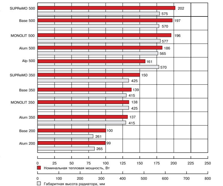
СРАВНЕНИЕ НОМИНАЛЬНОГО ТЕПЛОВОГО ПОТОКА И ГАБАРИТНОЙ ВЫСОТЫ СЕКЦИЙ РАДИАТОРОВ
