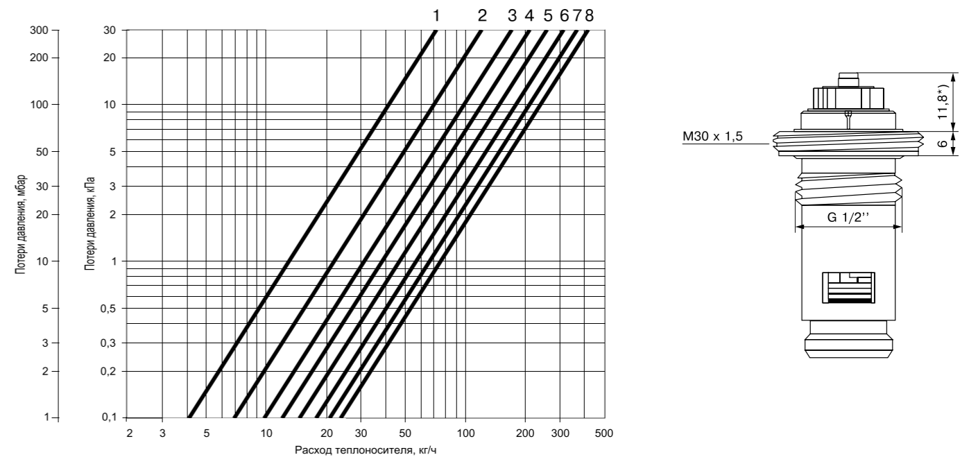
Диаграммы для термостатического клапана без узла нижнего подключения при 2 °С
